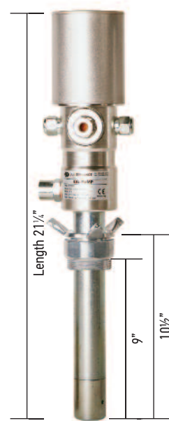
P/N 21100T-S2 5:1
