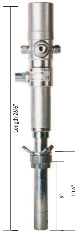
P/N 32091-S1 1:1
